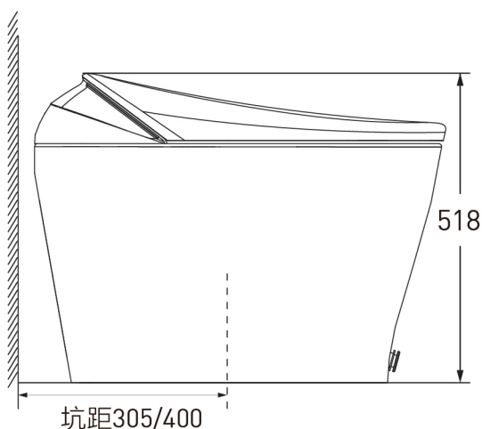
侧面图
