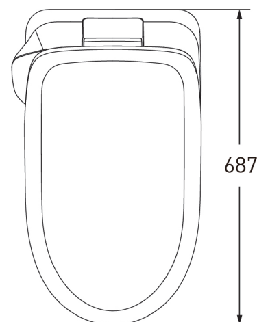
俯视图
