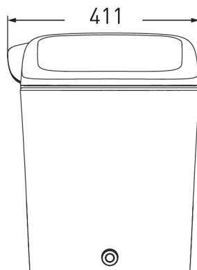
正视图
