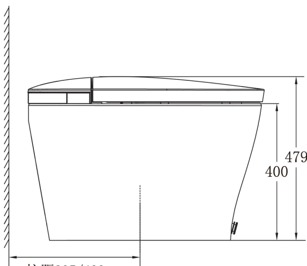
侧面图
