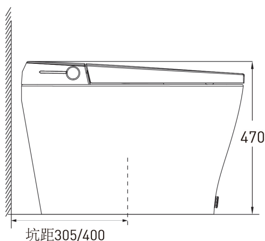
侧面图
