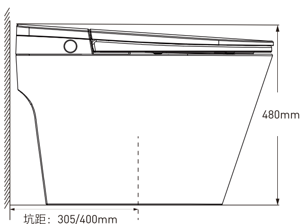
侧面图
